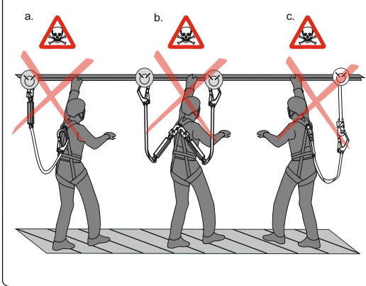
Рис. 10. Способы крепления стропов к анкерным устройствам
