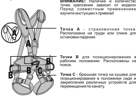
Рис. 5. Расположение и назначение крепежных точек на привязях
