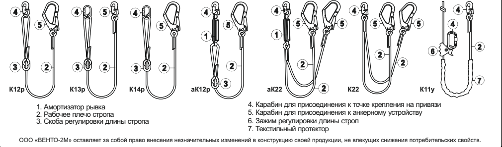
Рис. 6. Внешний вид, состав стропов
