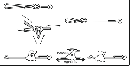
Рис. 5. Регулировка длины
