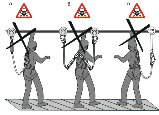
Рис. 9. Использование стропов без амортизатора.
